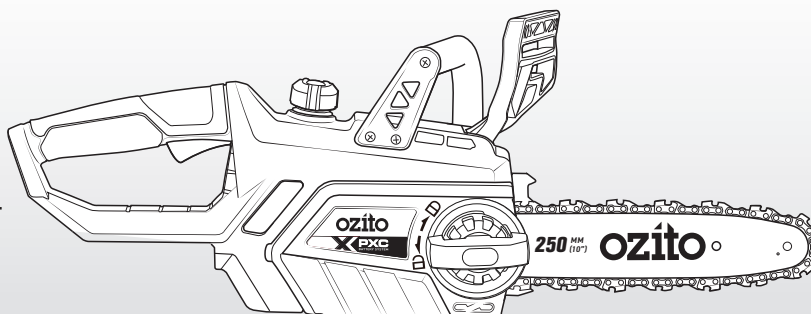
Guide Bar & Chain
