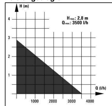
Leistungsdiagramm:
