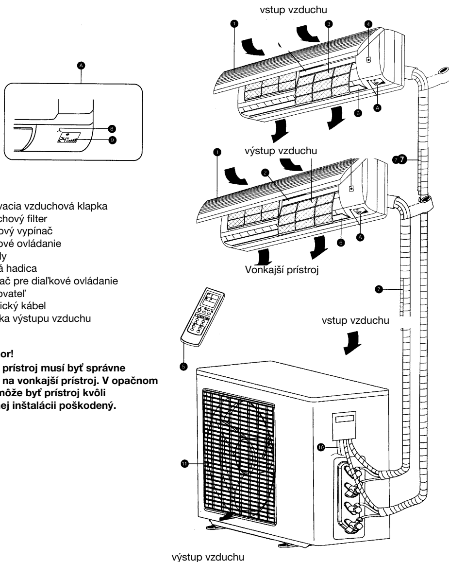
Vnútorný prístroj
