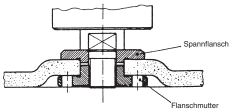
1 Anordnung der Flansche bei Verwendung einer gekröpften oder geraden Schleifscheibe
