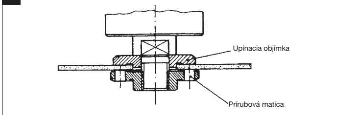
3 Usporiadanie príruby pri použití rovného rozbrusovacieho kotúča.
