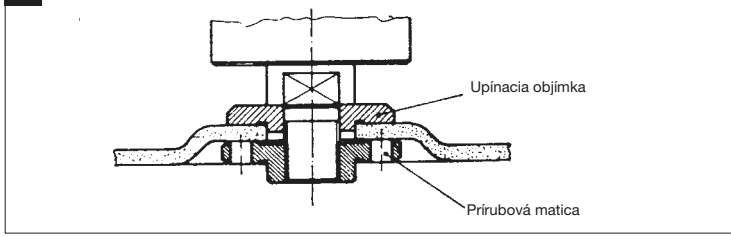
2 Usporiadanie príruby pri použití zalomeného rozbrusovacieho kotúča.
