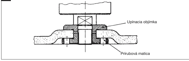
1 Usporiadanie príruby pri použití zalomeného alebo rovného brúsneho kotúča.
