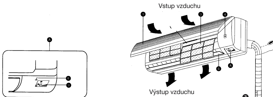
Vnitřní přístroj
