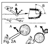
TENHA ATENÇÃO A: RECHAÇO DE ROTAÇÃO (Fig. 2A) A = Trajecto do rechaço B = Zona de reacção do rechaço
