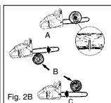
REACÇÕES DE EMBATE (RECHAÇO DE ENCRAVAMENTO) E TRACCÃO (Fig. 2B) A = puxar B = objectos fixos C = embater
