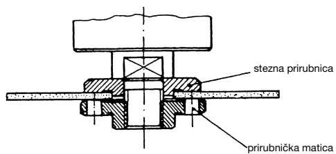
3 Raspored prirubnica pri upotrebi ravne rezne ploče
